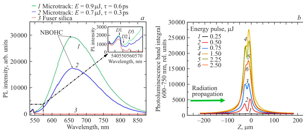
Рис. 2. (а) Спектры фотолюминесценции и КР двулучепреломляющих микротреков в плавленом кварце ( \Lambda = 1030 \text{ nm} , 100 \text{ kHz} , \tau = 0.3 \text{ ps} ). (б) Зависимость интеграла полосы 600–750 nm спектра фотолюминесценции от координаты вдоль микротрека.
