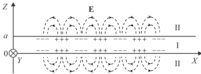
Рис. 1. Наноструктура „диэлектрик–проводник–диэлектрик“ (II — изолирующий слой, CL — проводящий слой). Штриховыми линиями показаны силовые линии напряженности электрического поля.
