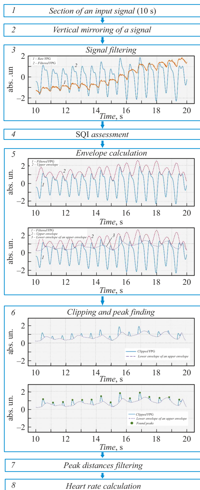
Рис. 3. Визуальное представление используемого алгоритма расчета ЧСС. 1 — входными данными является участок сигнала в 10 s; 2 — вертикальное отражение сигнала; 3 — фильтрация сигнала; 4 — оценка качества сигнала; 5 — построение огибающих; 6 — отсечение сигнала и поиск пиков; 7 — фильтрация расстояний между пиками; 8 — расчет ЧСС.
