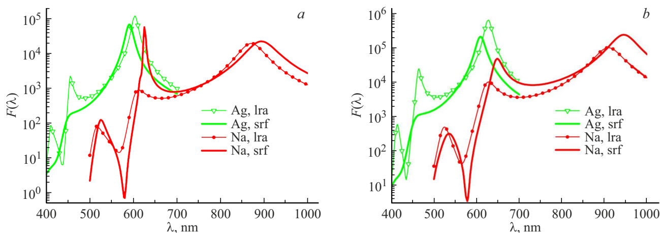
Рис. 2. Значения коэффициента усиления поля (10) в парных серебряных и натриевых частицах с различными зазорами, расположенных в среде \text{SiO}_2 : \delta = 2 (a), 1 nm (b). Приведены результаты, полученные с помощью локального (lra) и мезоскопического (srf) подходов.
