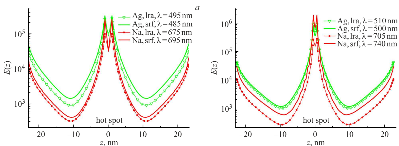
Рис. 3. Распределение интенсивности поля (9) вдоль образующих сфероидов в локальном (lra) и мезоскопическом (srf) случаях, вычисленное для пар серебряных и натриевых сфероидов с различными зазорами, расположенных в воздухе: \delta = 2 (a), 1 nm (b).
