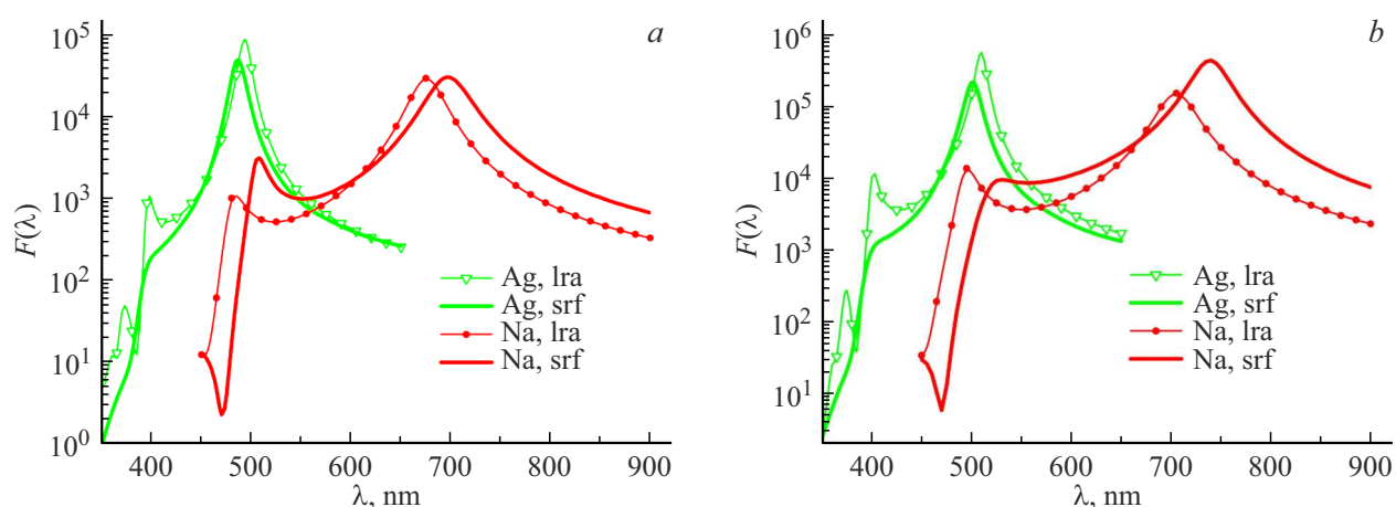
Рис. 1. Сравнение локального (lra) и мезоскопического (srf) подходов для пар серебряных и натриевых сфероидов с различными зазорами, расположенных в воздухе, при расчете коэффициента усиления поля (10) в центре зазора: \delta = 2 (a), 1 nm (b).
