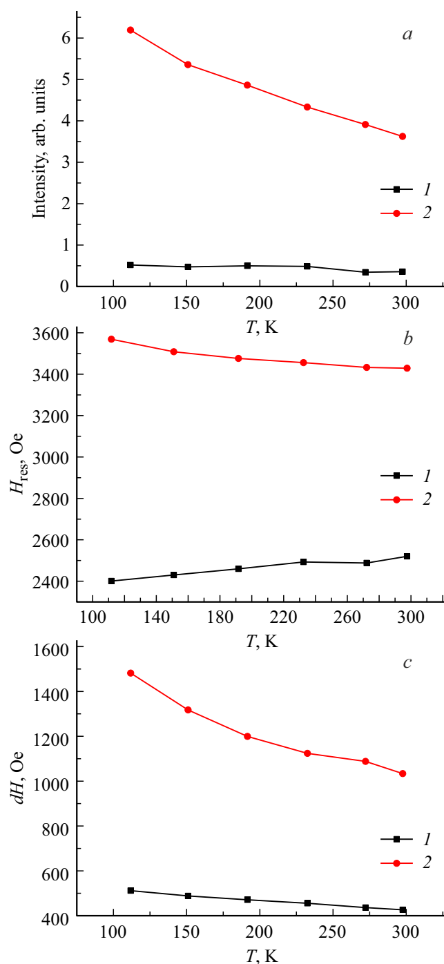
Рис. 5. Температурные зависимости: a — интенсивности, b — резонансного поля H_{\text{res}} , c — ширины линии dH ЭПР-сигнала на частоте \nu = 9\text{ GHz} в \text{LiMgFe}_2\text{V}_3\text{O}_{12} .
