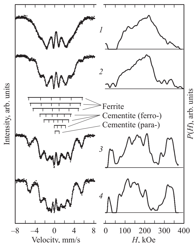
Рис. 2. Мёссбауэровские спектры (слева) и соответствующие им функции P(H) (справа) сплава Cr10Si3 после: 1 — МС и отжига при температурах T_{\text{ann}} : 2 — 500^\circ\text{C} , 3 — 600^\circ\text{C} , 4 — 800^\circ\text{C} . Температура измерений T = -196^\circ\text{C} .
