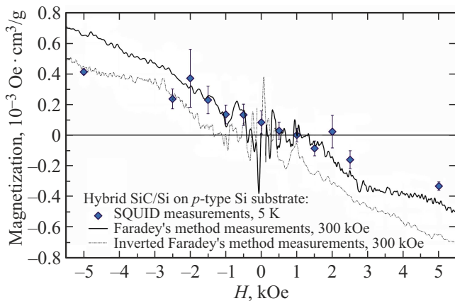
Рис. 4. Полевая зависимость намагниченности гибридной структуры SiC/Si, выращенной на поверхности кремния p -типа, полученная методом Фарадея при температуре 300 K в сравнении с результатами измерений на установке SQUID.
