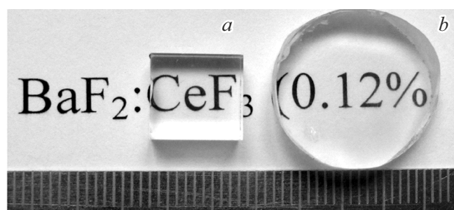
Рис. 1. Внешний вид исследованных образцов монокристалла (a) и керамики (b) BaF_2:Ce^{3+} .
