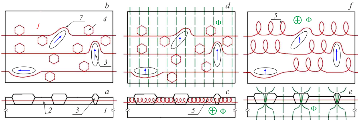
Рис. 4. Схематическое изображение транспорта носителей заряда в образце без магнитного поля ( a,b ) и с ориентацией вектора B вдоль ( c,d ) либо перпендикулярно ( e,f ) плоскости углеродного подслоя. 1 — подложка, 2 — проводящий подслоя наногрфита, 3 — островки VGN фазы с кластерами парамагнитных центров (дефектов), 4 — самопересекающиеся траектории носителей, обеспечивающие вклад в проводимость от механизма WL, 5 — движение носителей под действием силы Лоренца, 7 — траектории, огибающие островки VGN фазы. Магнитный поток \Phi обозначен зелеными линиями, линии тока j — красными линиями, синие стрелки ( b ) внутри островков VGN фазы (3) указывают магнитные моменты M от кластеров, обогащенных парамагнитными центрами в островках.
