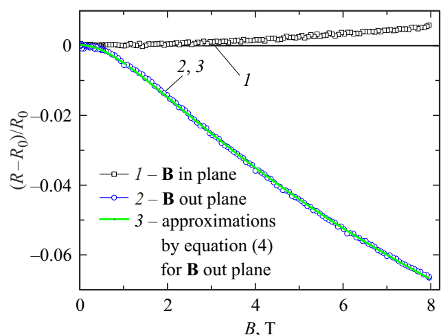
Рис. 3. Полевая зависимость относительного магнитосопротивления MR(B) для продольной (1) и перпендикулярной (2) ориентации магнитного поля относительно плоскости углеродного подслоя при температуре T = 7 К. Зеленая кривая (3) — аппроксимации уравнением (4) при перпендикулярной ориентации магнитного поля.
