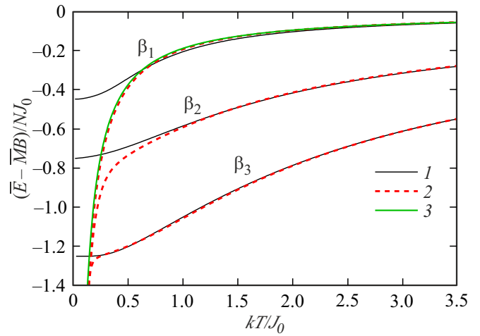
Рис. 5. Зависимость средней энергии спиновой цепочки от температуры в магнитных полях \beta_1 = 0, \beta_2 = 1, \beta_3 = 1.5 . 1 — точное решение, 2 формула (30), 3 приближенное аналитическое выражение (34).
