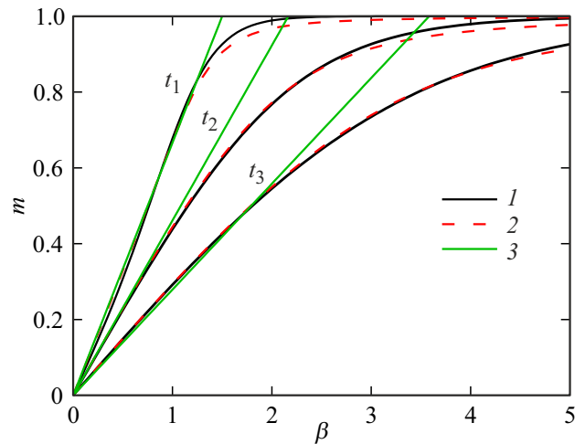
Рис. 3. Зависимость среднего магнитного момента от магнитного поля, посчитанная для трех различных значений температуры t_1 = 0.5 , t_2 = 1.5 и t_3 = 3.0 . Черная линия (кривая 1) посчитана по точному решению, красный пунктир (кривая 2) — формула (21), зеленая линия (кривая 3) — формула (22).
