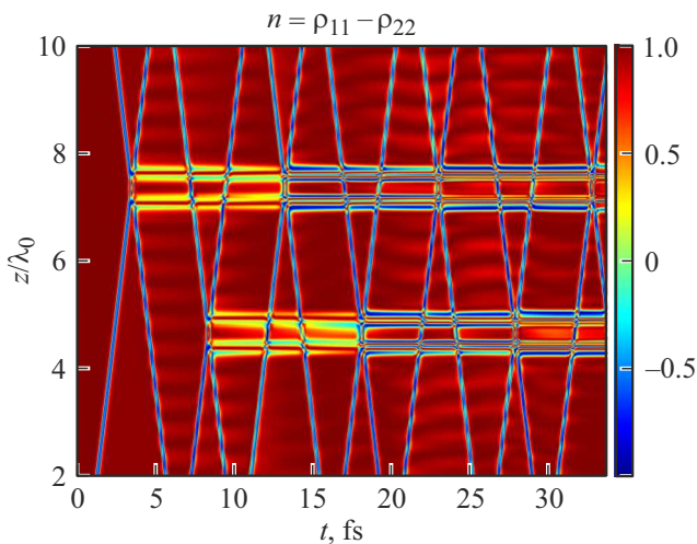
Рис. 2. (цветной онлайн). Пространственно-временная динамика разности населённости \rho_{11} - \rho_{22} двухуровневой среды.
