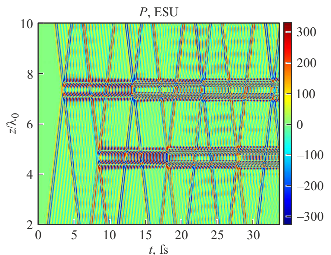
Рис. 3. (цветной онлайн). Пространственно-временная динамика поляризации двухуровневой среды P(z, t) .
