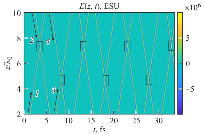
Рис. 1. (цветной онлайн). Схема распространения импульсов в среде. Цифрами отмечены первые 4 импульса. Направления распространения импульсов показаны стрелками. Каждое столкновение происходит в окрестностях точек z_{c1} \sim 4.3\lambda_0 и z_{c1} \sim 7.7\lambda_0 . Прямоугольники отмечают эти области.
