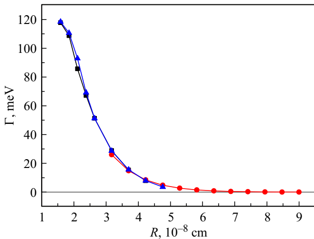
Рис. 2. Зависимость автоионизационной ширины от расстояния: ■ — данные из работы [14] для триплетного терма, ▲ — данные из работы [14] для синглетного терма, ● — экстраполяция данных в область больших расстояний с помощью экспоненциальной зависимости.
