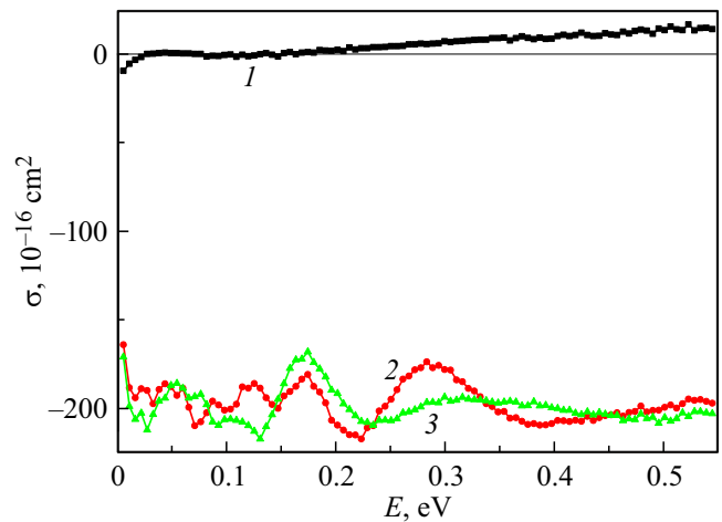
Рис. 3. Зависимость от энергии столкновения сечений сдвига частоты магнитного резонанса: 1 — сечение сдвига частоты ( \bar{\sigma}_{0,1} ), определяемое интерференцией амплитуд упругого рассеяния на синглетном ( s ) и триплетном ( t ) термах; 2 — сечение сдвига частоты ( \bar{\sigma}_{0,2} ), определяемое интерференцией амплитуд упругого рассеяния на синглетном ( s ) и квинтетном ( q ) термах; 3 — сечение сдвига частоты ( \bar{\sigma}_{1,2} ), определяемое интерференцией амплитуд упругого рассеяния на триплетном ( t ) и квинтетном ( q ) термах.
