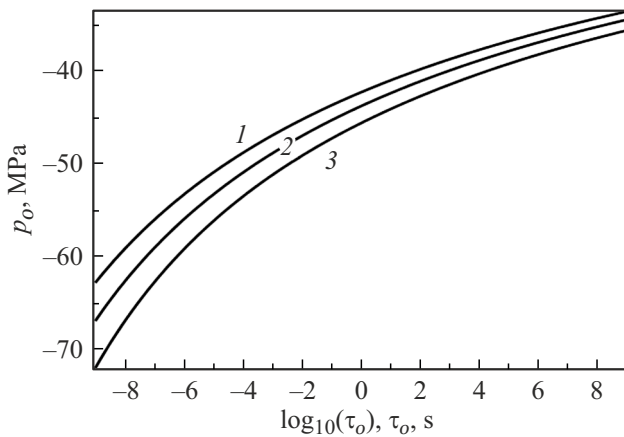
Рис. 3. Зависимость порогового давления гомогенной кавитации внутри масляной капли от времени ожидания при трех разных размерах капли (расчет по (13)). Расчетные данные [3]: T = 300 \text{ K} , \gamma_o = 23 \text{ mNm}^{-1} , \gamma_{ow} = 45 \text{ mNm}^{-1} , \delta_o = -0.116 \text{ nm} , \kappa_o = 5.4 \cdot 10^9 \text{ s}^{-1} \cdot \text{nm}^{-3} , N = 50 . 1 — R_o = 200 ; 2 — 100; 3 — 50 nm.
