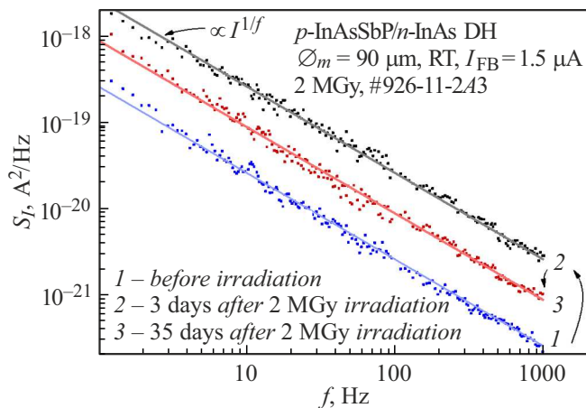
Рис. 7. Частотная зависимость токового шума S_I для диода \varnothing_m = 90 \mu\text{m} : 1 — до облучения, 2 — через три дня после облучения дозой 2 MGy, 3 — через 35 дней после окончания облучения. Прямые линии — значения функций вида S_I \propto 1/f .
