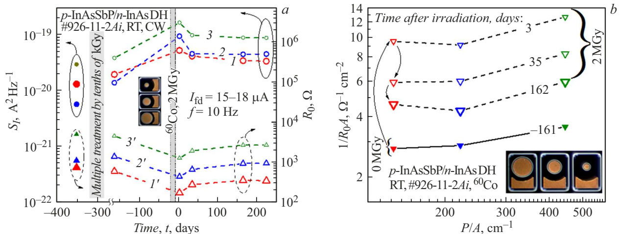
Рис. 5. a — зависимость величины шума (S_I)_{10 \text{ Hz}} и сопротивления (R_0) от времени, прошедшего после окончания облучения для трех BSI-диодов с диаметрами мез 90, 180 и 280 \mu\text{m} (кривые 1(1'), 2(2') и 3(3') соответственно), b — зависимость произведения R_0A (300 K) от соотношения периметра ( P ) и площади диодов ( A ) до и после облучения дозой 2 MGy в разные моменты времени.
