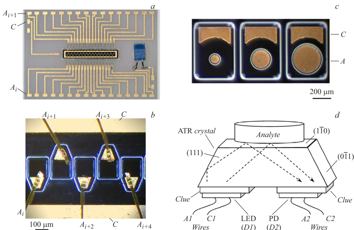
Рис. 1. a — общий вид диодной линейки 1 \times 32 , смонтированной на контактной плате, b — фотография ее фрагмента, на котором обозначены общий катод (C), 5 мез ( A_i ) с присоединенными к ним золотыми проволоками; c — фотография диодов с круглыми мезами ( \varnothing_m = 90, 180, 280 \mu\text{m} ) и широкими анодами (A); d — схема датчика с иммерсионным сопряжением диодов и кристалла МНПВО, где „ATR crystal“ — кристалл МНПВО, „Glue“ — оптический клей, „D1, D2“ — чипы диодов, „Wires“ — золотые провода, подсоединенные к анодам (A) и катодам диодов (C), „Analyte“ — анализируемое вещество, стрелки — примерный ход некоторых лучей, вышедших из СД (LED, D1), испытавших полное внутреннее отражение на ГР кристалл МНПВО/аналит и попавших в поглощающий слой ФД (PD, D2). Схема не в масштабе.
