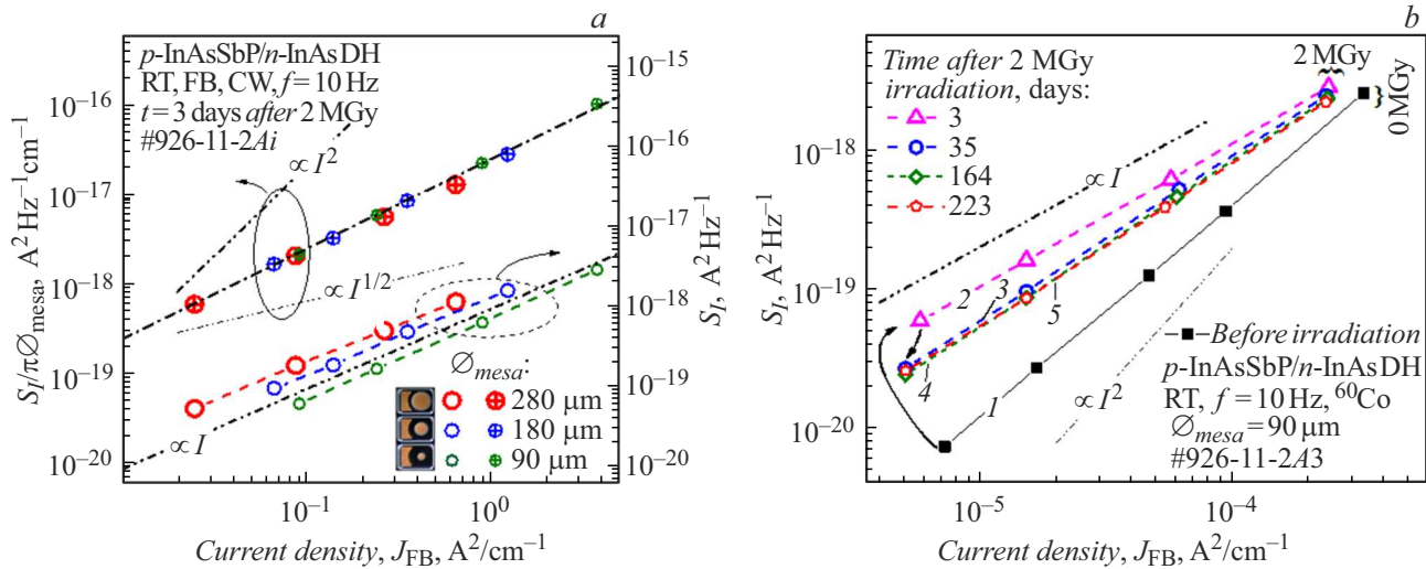
Рис. 6. a — зависимость шума S_I (правая шкала) и нормированного на периметр шума S_I / \pi \varnothing_m (левая шкала) от плотности прямого тока в диодах с \varnothing_m = 90, 180 и 280 \mu\text{m} через три дня после окончания облучения дозой 2 MGy; b — зависимость шума от прямого тока в образце \varnothing_m = 90 \mu\text{m} до (сплошные символы, кривая 1) и после облучения („пустые“ символы) через 3, 35, 164 и 223 дня (кривые 2–5 соответственно) после его окончания при температуре 25 °C–29 °C.
