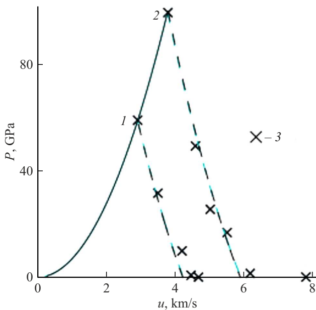
Рис. 4. Давление ( P ) как функция массовой скорости ( u ) на ударной адиабате (сплошная линия) и изэнтропах разгрузки (штриховые линии) ударно-сжатых образцов никеля начальной пористости m = 2.305 при \alpha = 1 (черные линии) и 0.5 (голубые линии). Экспериментальные данные: 3 — [62]. В точке 1 — u = 2.91 km/s, P = 59 GPa, в точке 2 — u = 3.78 km/s, P = 99.4 GPa.
