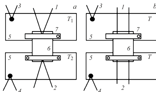
Рис. 3. а — схема измерения коэффициента Зеебека; 1, 2 — измерительные термопары; 3, 4 — термопары, контролирующие температуру нагревательных столиков 5; 6 — образец; 7 — графитовые прижимы; б — схема измерения удельного сопротивления; 1, 2 — измерительные провода.
