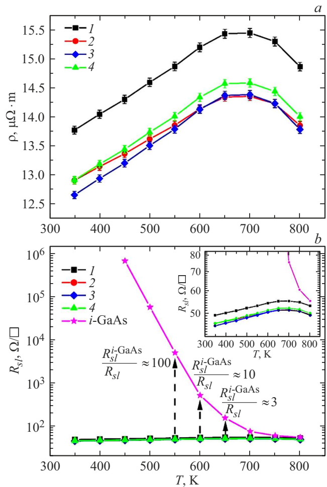
Рис. 5. a — экспериментальная температурная зависимость удельного сопротивления исследованных образцов, b — сопоставление слоевого сопротивления образцов и подложки полуизолирующего арсенида галлия.
