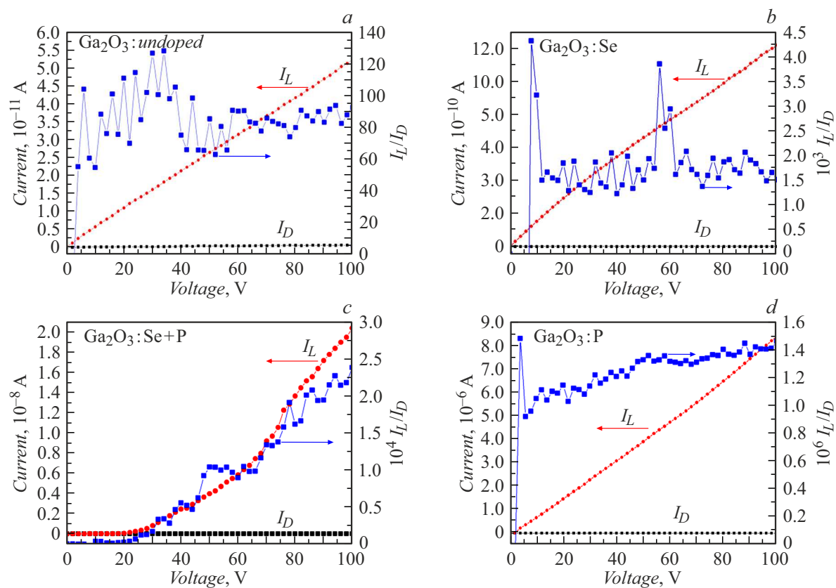
Рис. 4. Темновые и световые ВАХ образцов с нелегированной (а) и легированными пленками оксида галлия (b–d); \lambda = 254 nm; I_D — темновой ток; I_L — ток во время действия излучения.
