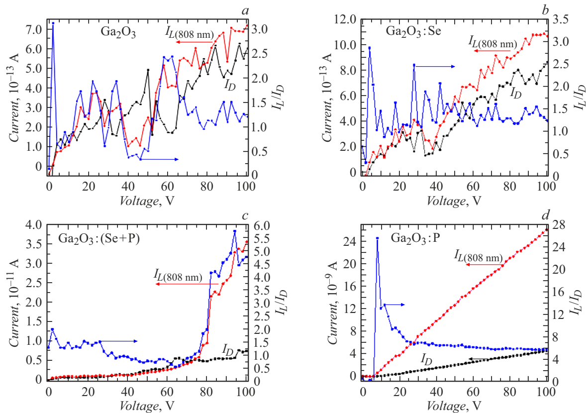
Рис. 6. Темновые и световые ВАХ образцов с нелегированной (а) и легированными пленками оксида галлия (b–d); \lambda = 808 nm.
